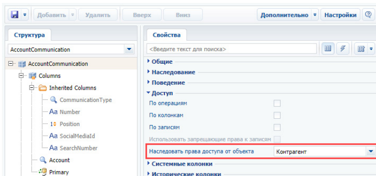
Рис. 600 — Настройка наследования прав доступа от родительского объекта
