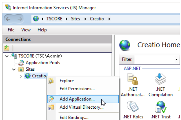
Рис. 685 — Выбор команды добавления приложения в IIS
