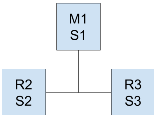
Рис. 703 — Конфигурация "трех узлов": quorum = 2
