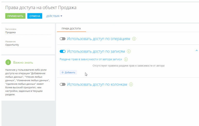
Рис. 609 — Пример добавления ролей для настройки прав доступа
