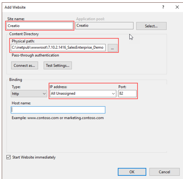
Рис. 684 — Окно параметров нового сайта
