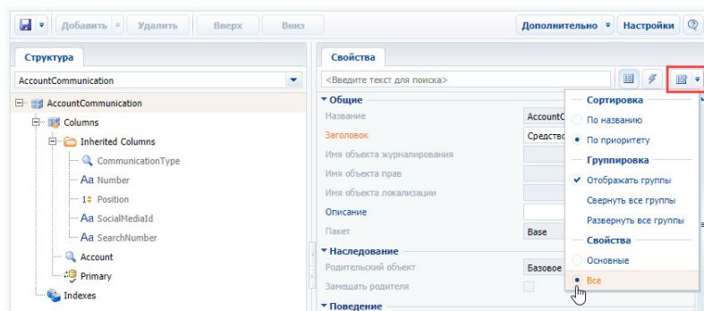
Рис. 599 — Переход в расширенный режим отображения свойств объекта
